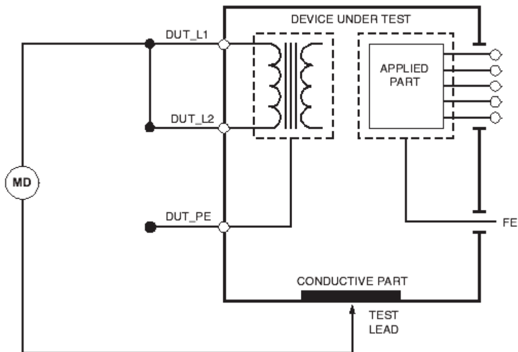
o‘lchash sxemasi.
